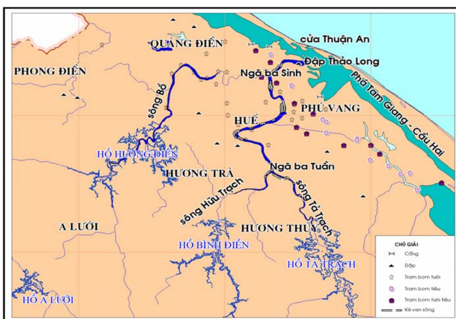
Một số công trình khai thác, sử dụng nước chủ yếu trên sông Hương
