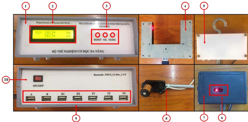
Hình 7. Hệ thiết bị thí nghiệm cơ học hoàn chỉnh
