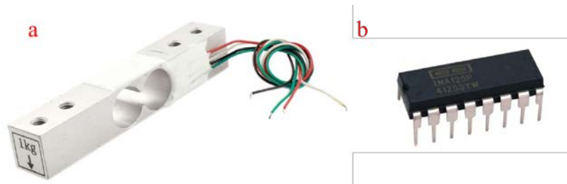
Hình 5. (a) Cảm biến lực YZC131-1kg; (b) Mạch khuếch đại vi sai INA125P
